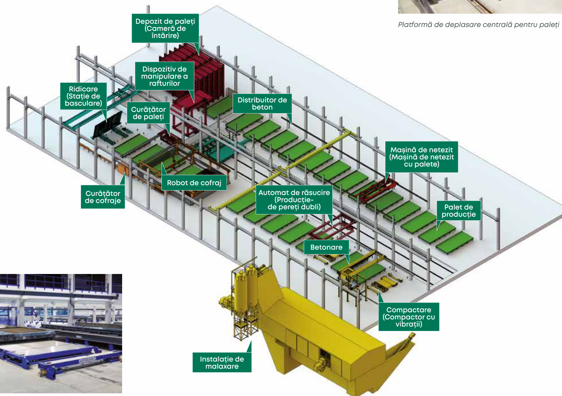
Compactare (Compactor cu vibrații)
